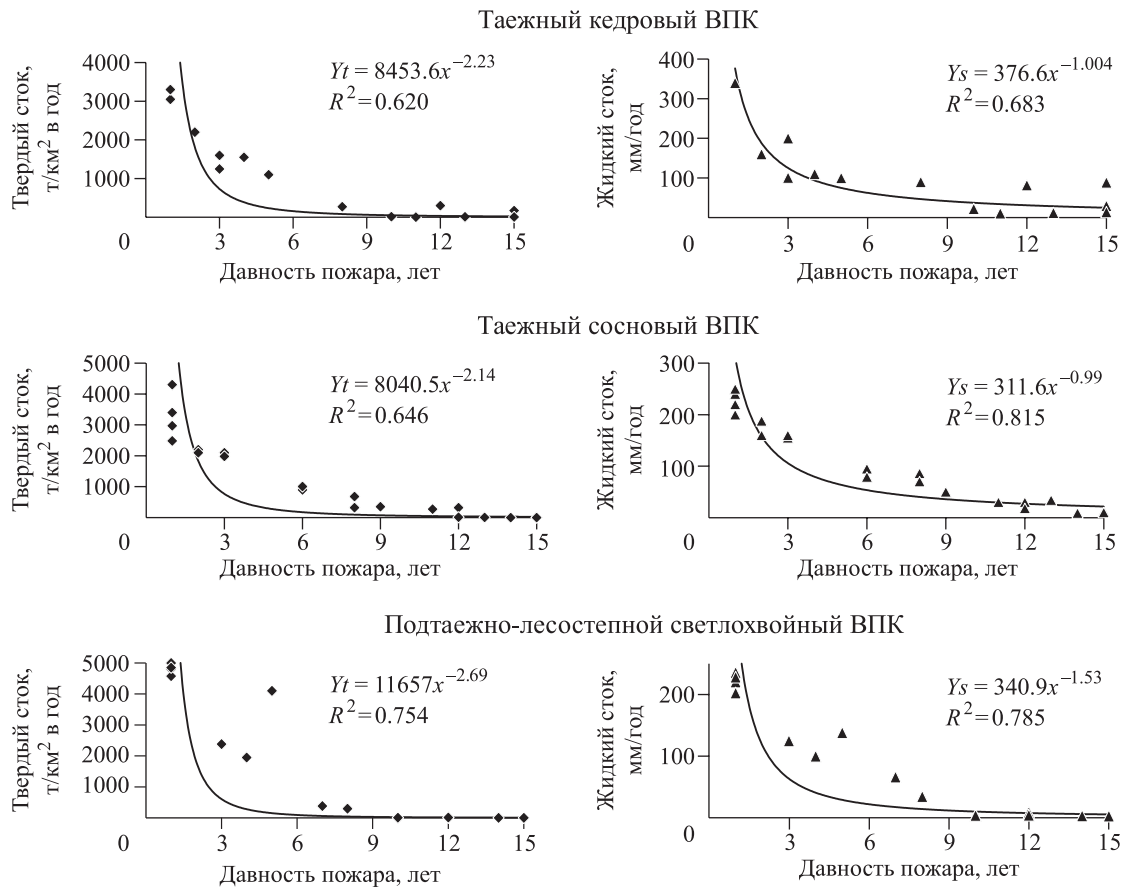
Рис. 2. Зависимость изменения поверхностного твердого и жидкого стока от давности пожаров в таежном кедровом, сосновом и подтаежно-лесостепном светлохвойном ВПК.
