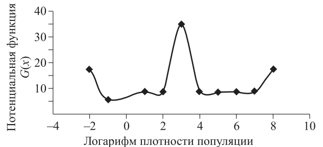
Рис. 5. Эмпирическая функция состояния G(\ln x) популяции сибирского шелкопряда на Ангаре в 1953–1969 гг.
