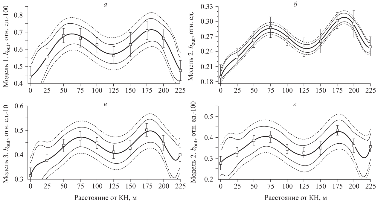
Рис. 1. Зависимости коэффициента b_{out} от расстояния до края естественных насаждений с указанием границ доверительных интервалов для линии регрессии и разброса значений, а также стандартных ошибок b_{out} отдельных моделей.
